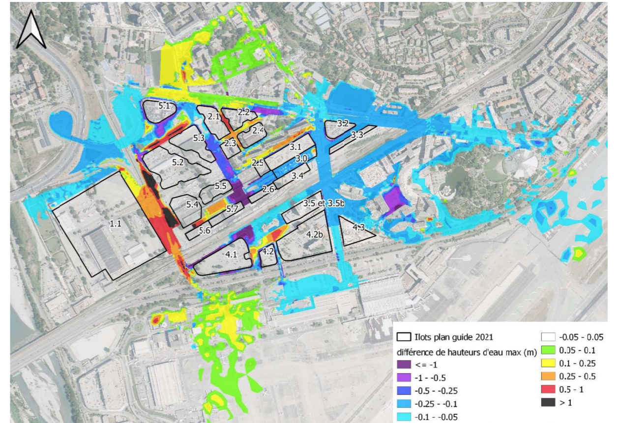
Figure 31 : Différence de hauteur d'eau maximales entre C3A et Réf2
