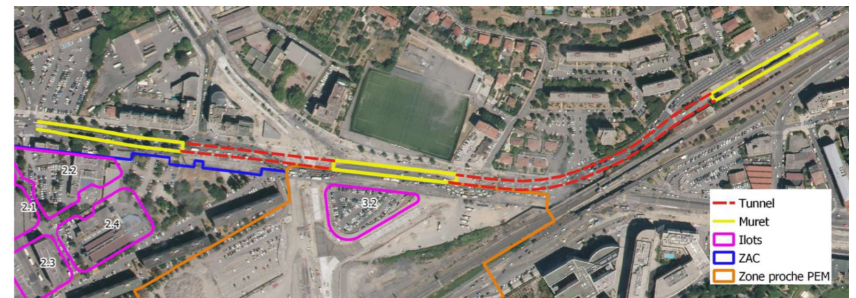
Figure 6 : Localisation des tranchées couvertes et ouvertures de la SOVM phase 1
