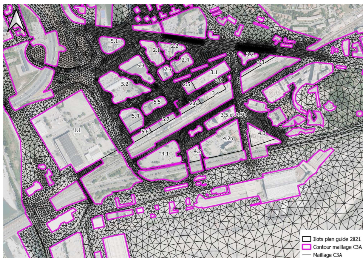
Figure 20 : Maillage du modèle C3A
