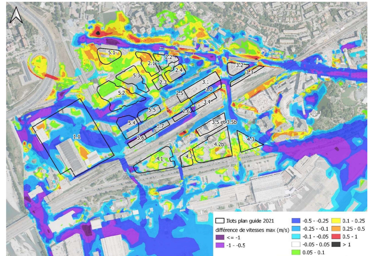
Figure 49 : Zoom sur la ZAC du Grand Arénas de la différence de vitesse d'écoulement maximale entre C1A et C1
